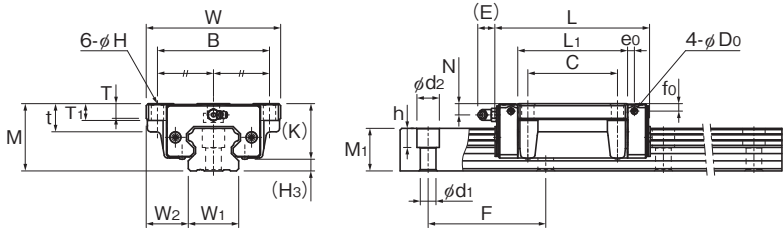
HSR45~85CB/HB/XCB/XHB型
