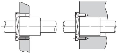
僅通過一個法蘭安裝
