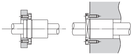
通過套管安裝的軸襯套
