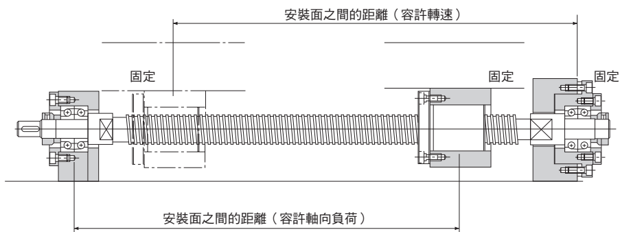
圖10 螺桿安裝方法:固定-固定
