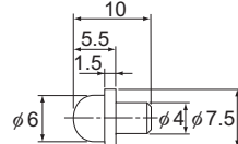
PB1021B
