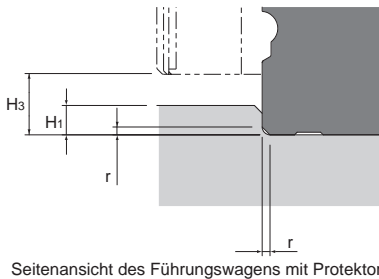
Seitenansicht des Führungswagens mit Protector
