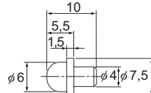
Ausführung PB1021B
