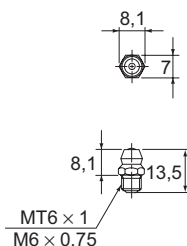
Ausführung A-MT6 × 1 (MT6 × 1) Ausführung A-M6F (M6 × 0,75)
