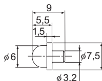
Ausführung NP3,2 × 3,5
