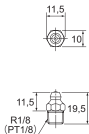
Ausführung A-PT1/8
