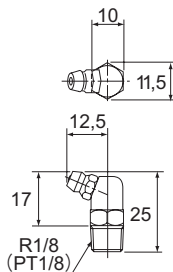
Ausführung B-PT1/8
