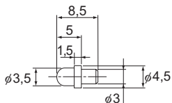
Ausführung PB107
