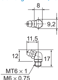
Ausführung B-MT6 × 1 (MT6 × 1) Ausführung B-M6F (M6 × 0,75)
