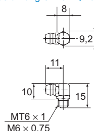
Ausführung C-MT6 × 1 (MT6 × 1) Ausführung C-M6F (M6 × 0,75)
