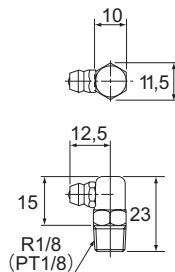
Ausführung C-PT1/8
