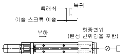
그림11 백래쉬
