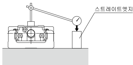
그림8 주행평행도
