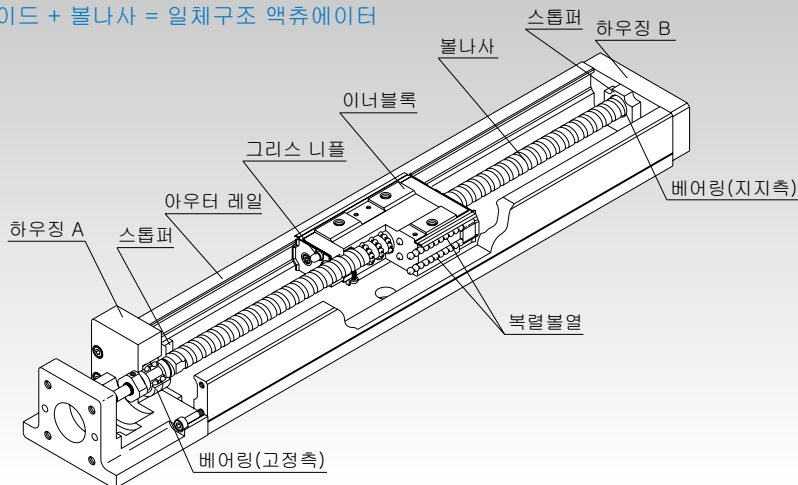
그림1 LM 가이드 액추에이터 KR형의 구조
