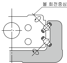
그림4 SKR형의 접촉구조
