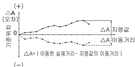
그림7 위치결정정도
