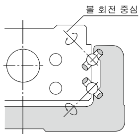
그림4 KR형의 접촉구조
