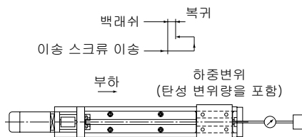
그림9 백래쉬
