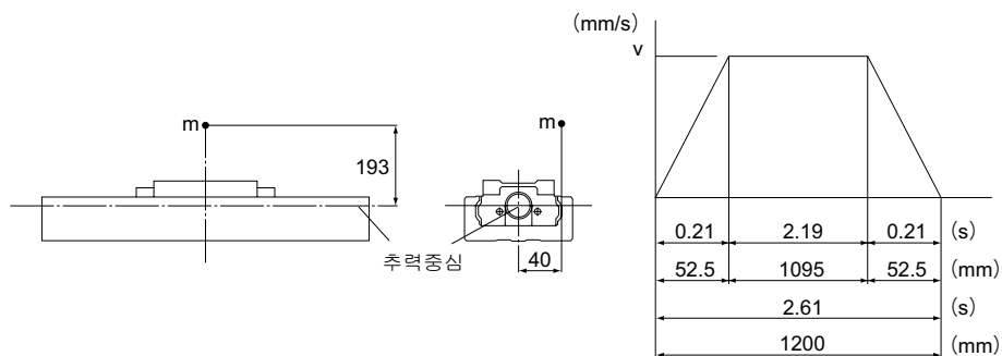
그림1 속도선도
