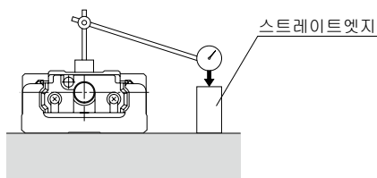
그림10 주행평행도
