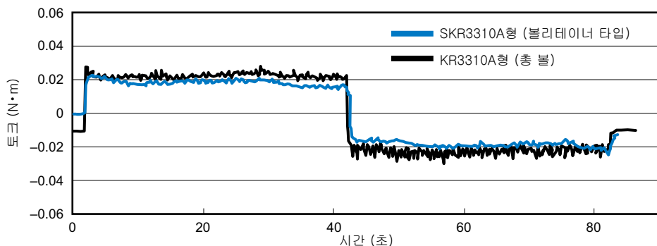
그림6 SKR형과 KR형의 토크 변동치 비교
