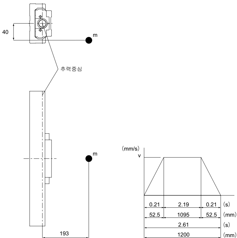
그림2 속도선도
