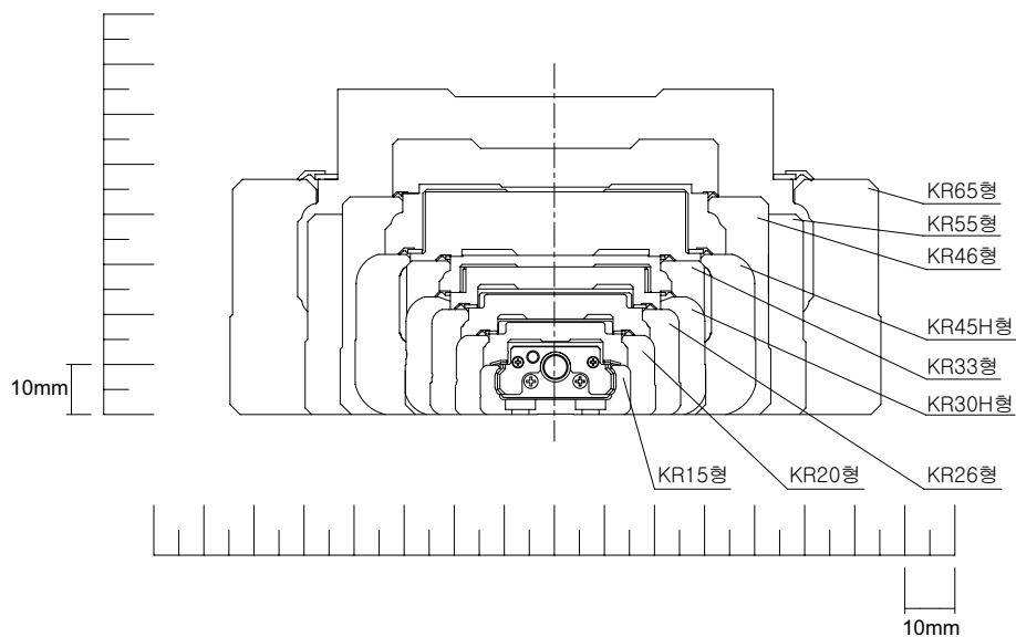
그림5 단면형상도
