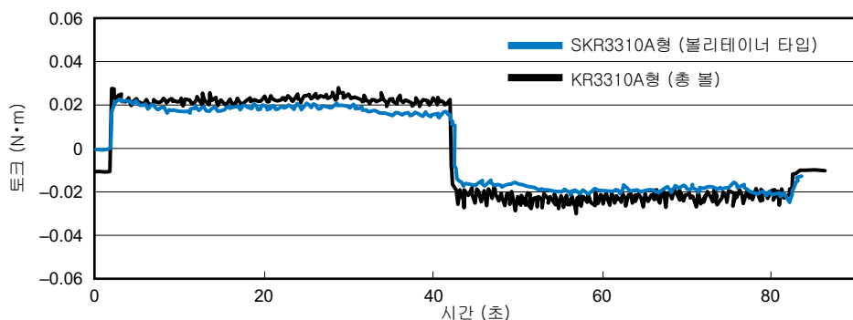
그림5 SKR형과 KR형의 토크 변동치 비교
