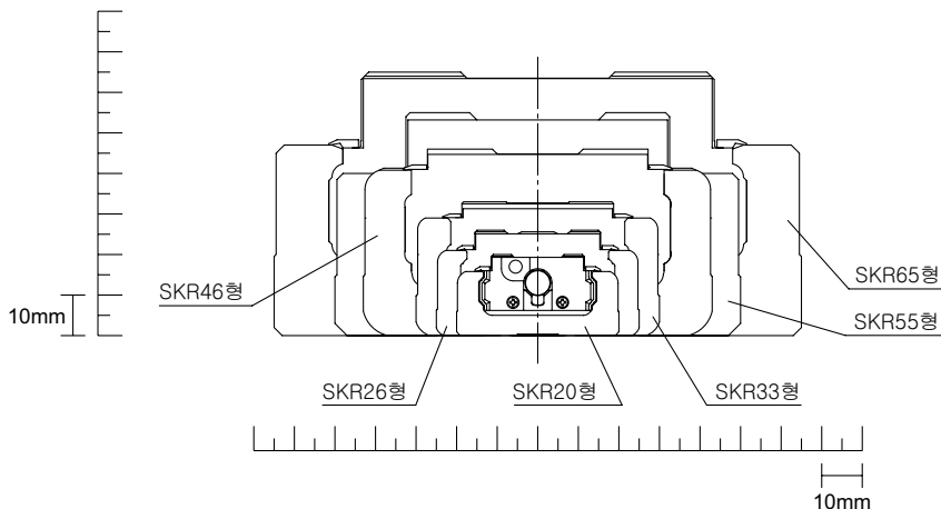
그림5 단면 형상도
