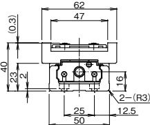
B-B 단면
