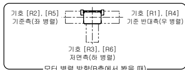
【모터 병렬의 경우】
