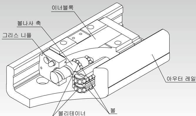
그림1 볼리테이너 타입 LM 가이드 액추에이터 SKR형의 구조
