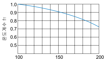
그림1 온도계수 ( f_t )
