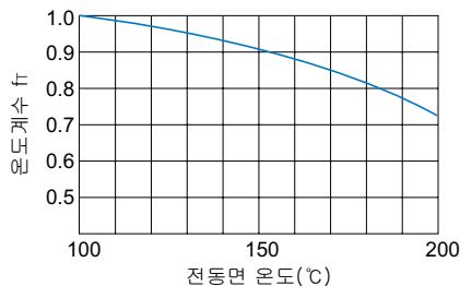
그림1 온도계수 ( f_t )
