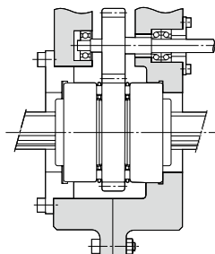
그림2 스플라인 너트의 장착예
