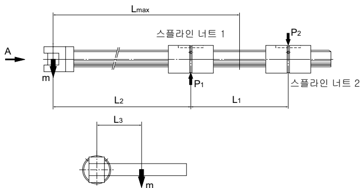
A에서 볼 그림5
