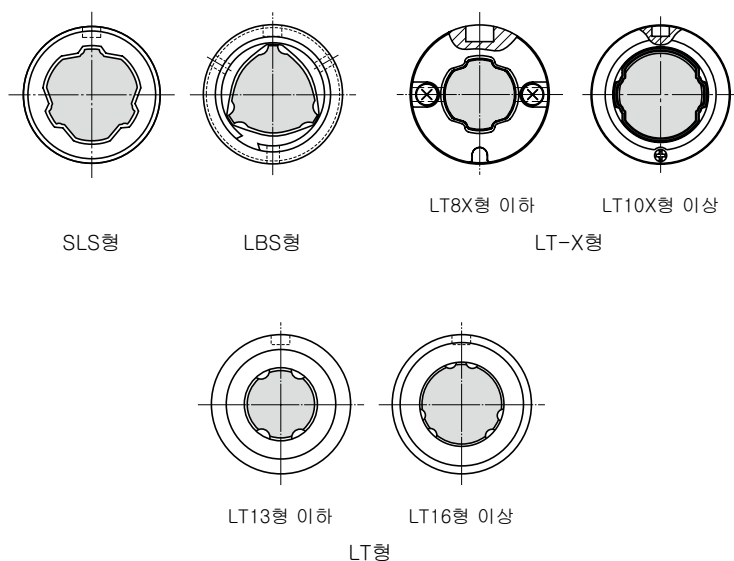
그림1 키홈의 위치
