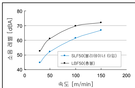
소음레벨 비교
