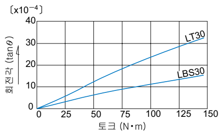
그림8 CL 클리어런스시의 LBS형과 LT형의 비교
