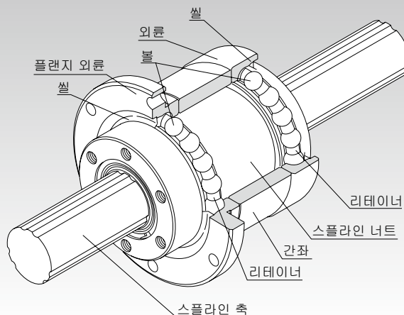
그림1 로터리 볼스플라인 LTR형의 구조
