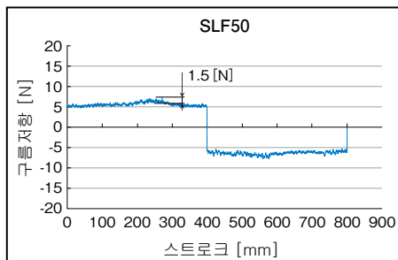
구름저항시험
