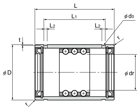
ST...UU형 (輕하중용)
