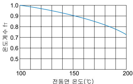
그림3 온도계수 ( f_T )
