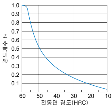
그림2 경도계수 ( f_H )
