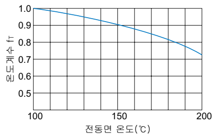
그림3 온도계수 ( f_T )
