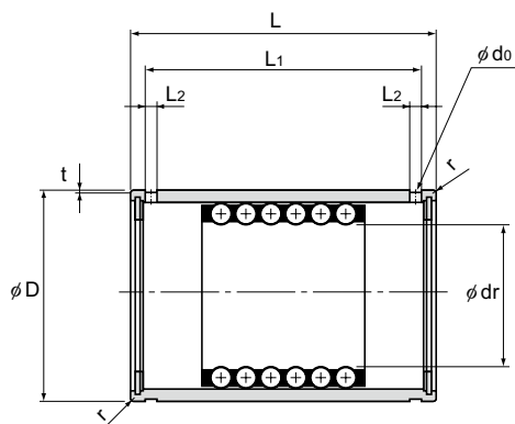
ST-B형 (中하중용)
