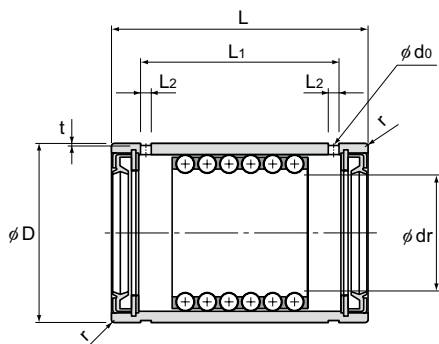
ST...UUB형 (中하중용)
