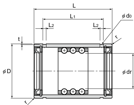
ST...UU형 (輕하중용)
