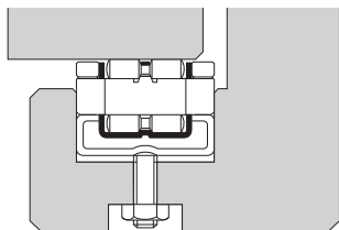
(a) 전용 스프링패드 의한 방법
