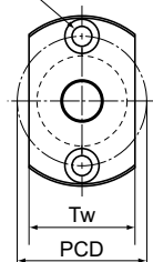
너트 타입I
