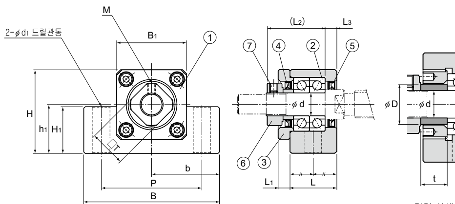
EK 10~20형
