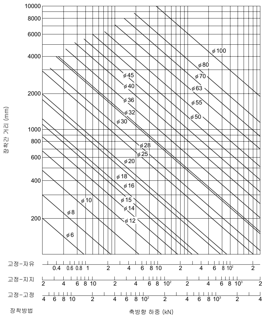
그림12 허용 축방향 하중선도
