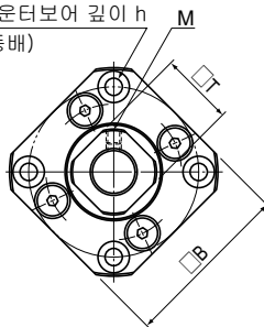
FK 10~30형
