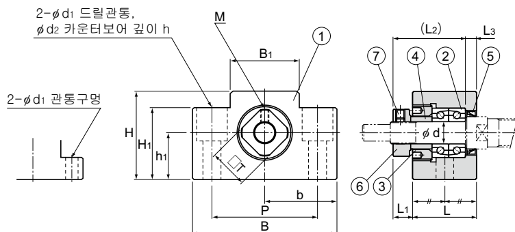
EK 4, 5형
