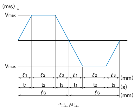
속도선도
