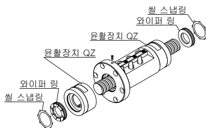
윤활장치 QZ+와이퍼 링
