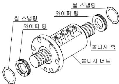
외관도
