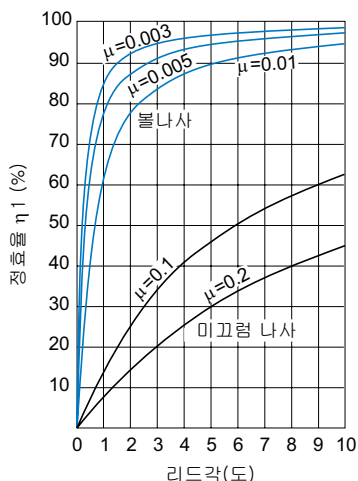
그림1 정효율(회전→직선)
