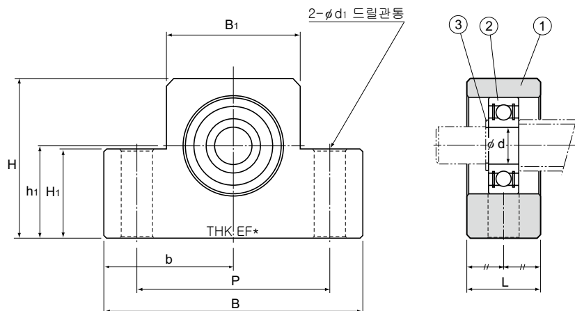
EF 10~20형
