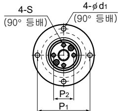
볼나사 부 (0812A, 1015A형)
