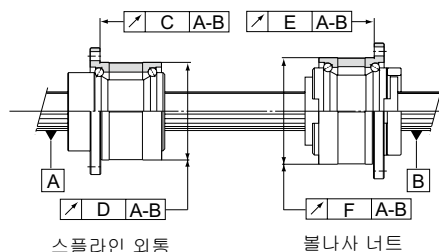
BNS형
