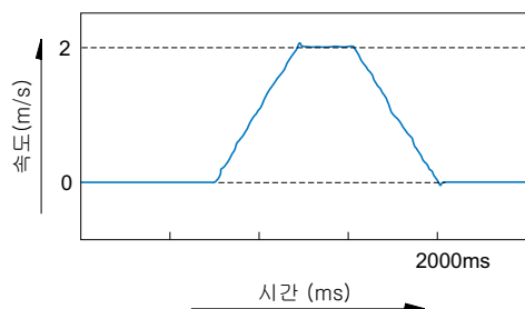
그림7 속도선도
