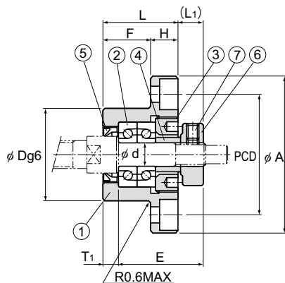
장착방법 A
