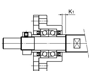
FK형
