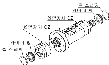
윤활장치 QZ+와이퍼 링
