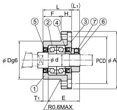
장착방법 A
