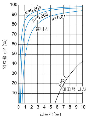
그림2 역효율(직선→회전)
