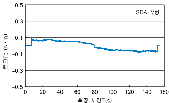
그림3 토크 변동 데이터
