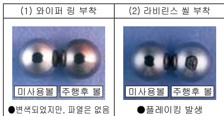
2000km 주행후 볼의 변화
