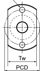
너트 타입II
