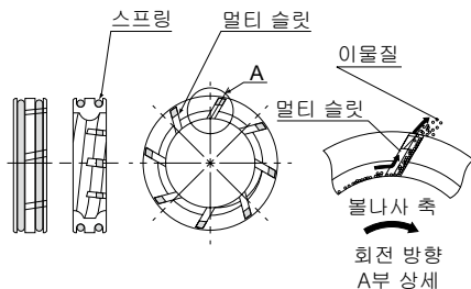
구조도
