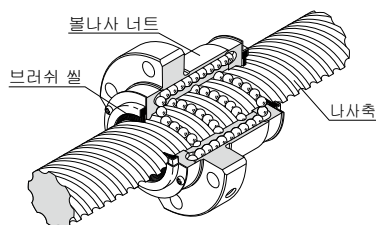
브러쉬 씰
