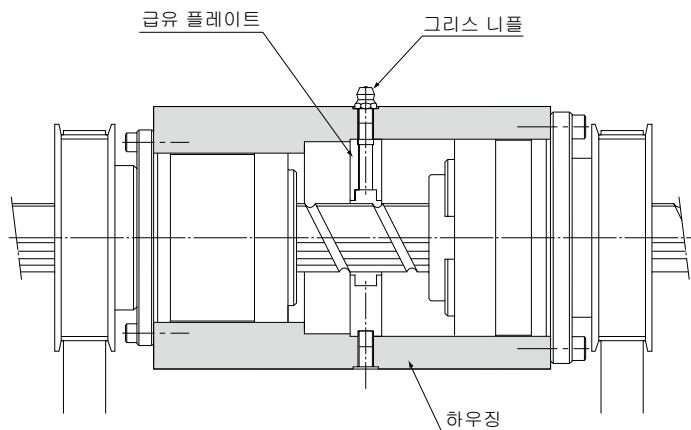
그림6 윤활 방법
