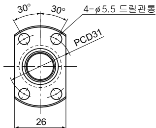
X-X 단면
