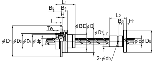
볼나사 부 (0812A, 1015A형)
