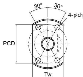
너트 타입 II
