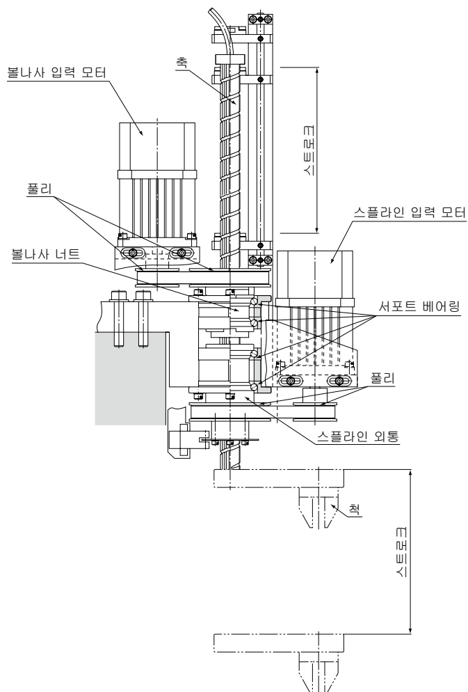
그림5 BNS형의 사용예
