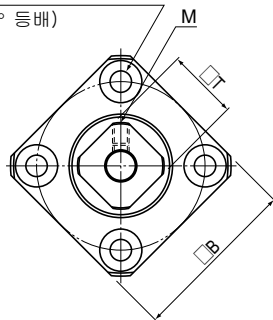
FK 4~8형
