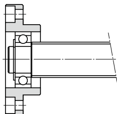
FF형
