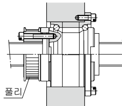
플랜지 역방향
