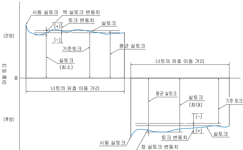
그림7 예압 토크 용어
