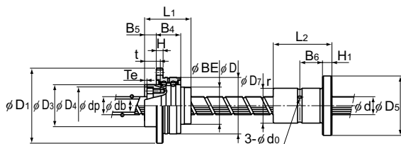
볼나사 부 (1616A~4040A형)
