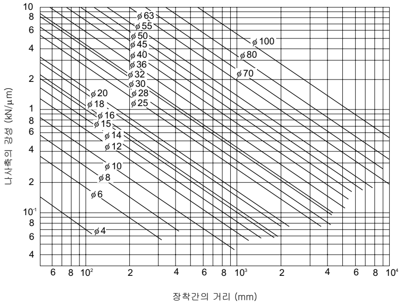
그림15 너트축의 축방향 강성(고정-고정)
