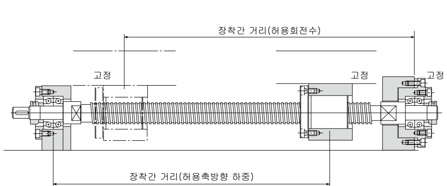
그림3 나사축의 장착방법: 고정-고정
