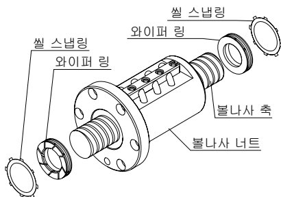
외관도
