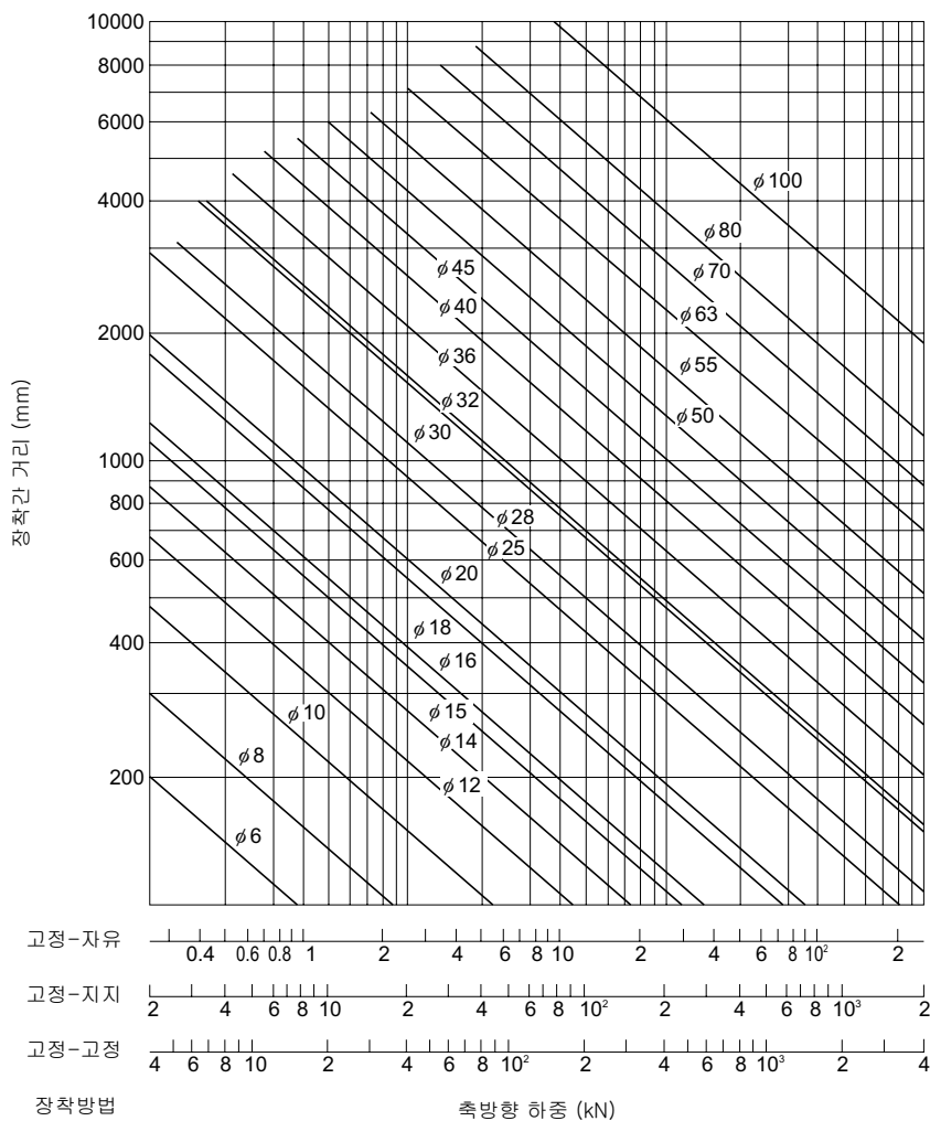
그림5 허용 축방향 하중선도
