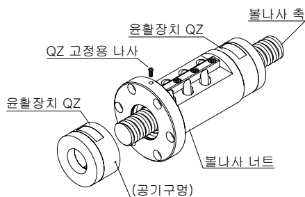
윤활장치 QZ
