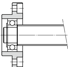
EF형
