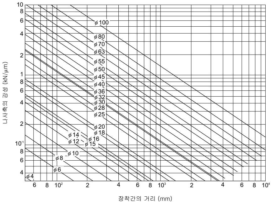
그림14 나사축의 축방향 강성(고정-자유, 고정-지지)
