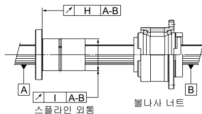
NS형
