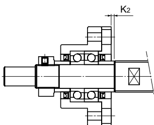
FK형
