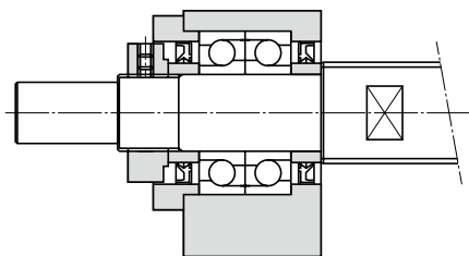
BK형
