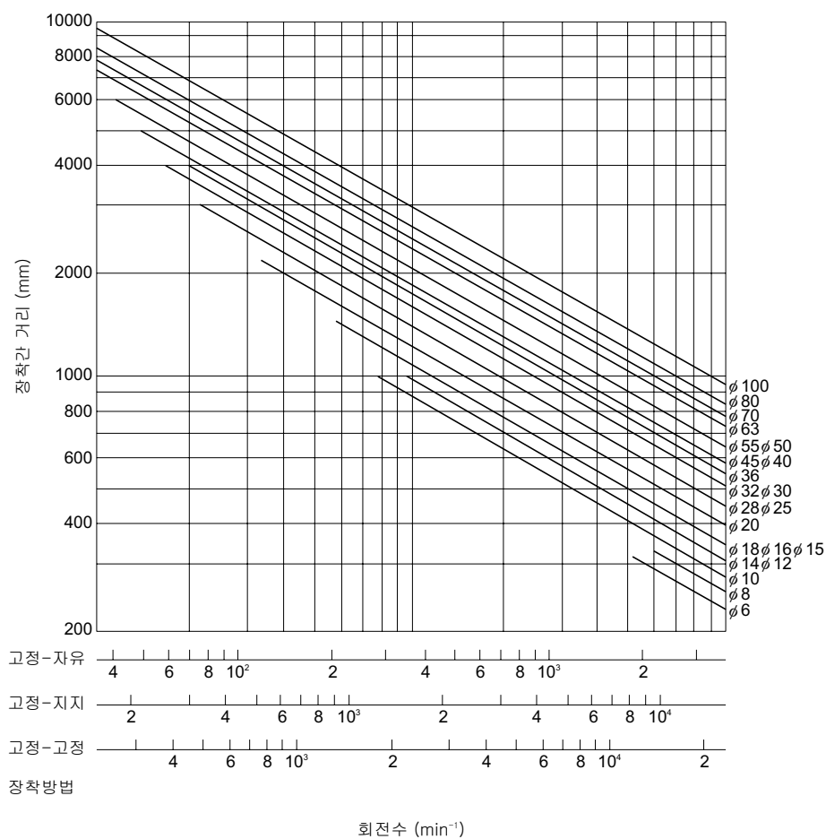
그림13 허용회전수 선도
