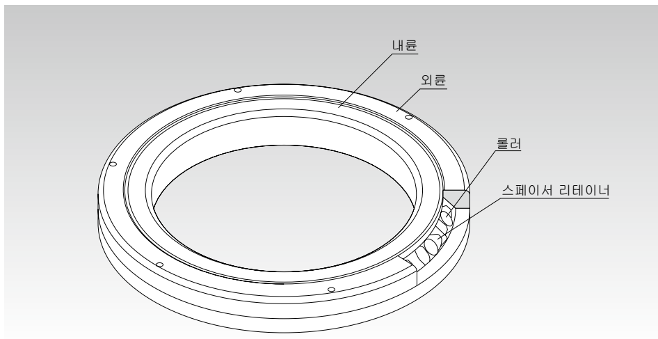
그림1 크로스 롤러링 RB형의 구조
