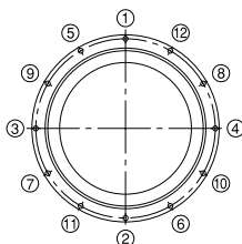
그림1 체결 순서
