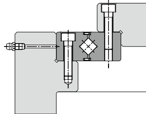
e. 선회부 내·외륜 동일방향 체결 (섀 부착)
