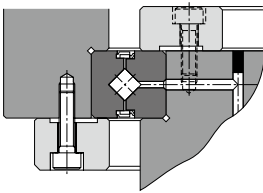
a. 선회부 외륜회전 내·외륜 체결후 본체 중량물을 조립하는 예
