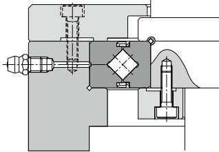
b. 선회부 내륜 회전 (섀 부착)
