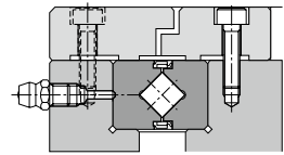
c. 선회부 내·외륜 동일방향 체결 (섀 부착)
