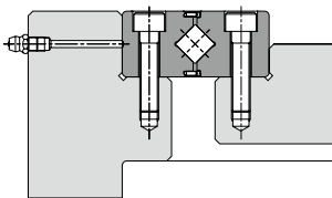
d. 선회부 내·외륜 동일방향 체결 (섀 부착)
