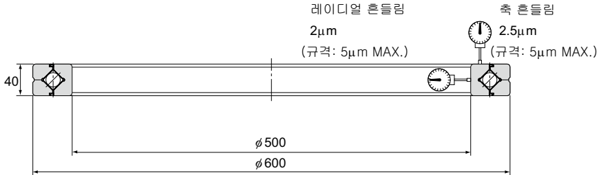
RB50040CC0USP형의 내륜 회전 정도
