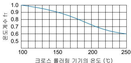
그림1 온도계수 ( f_T )
