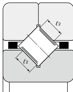
철판 리테이너 부착(종래품)
