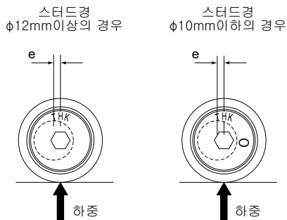
그림2 편심방향 위치관계
