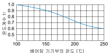
그림1 온도계수 ( f_r )
