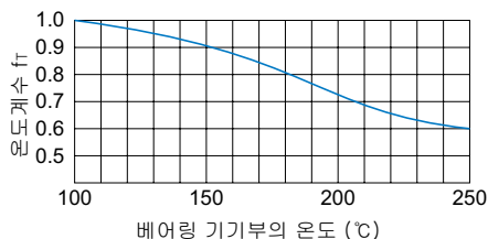
그림1 온도계수 ( f_r )
