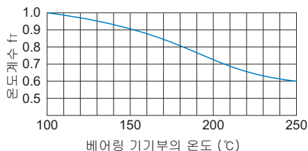
그림1 온도계수 (f t )
