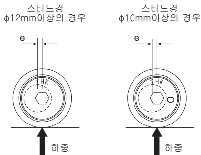
그림2 편심방향 위치관계
