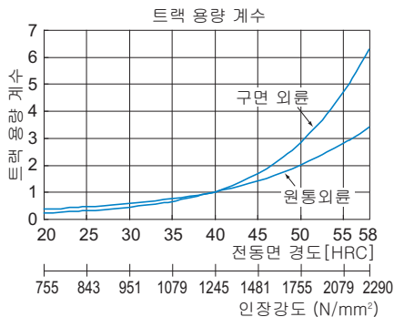
그림2 트랙 용량 계수
