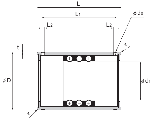
ST형 (輕히중용)
