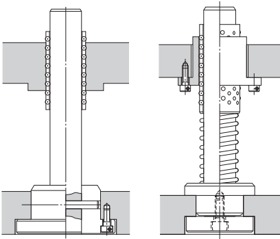
그림2 장착예
