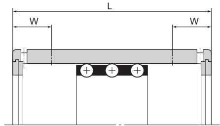
그림4 외통의 측정범위
