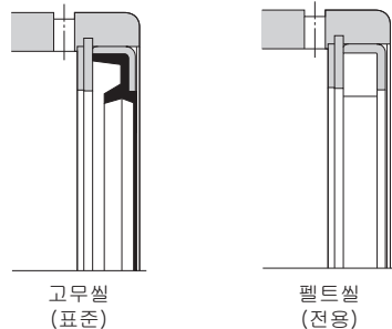
그림1 LM 스트로크용 씰의 종류
