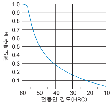
그림2 경도계수 ( f_H )
