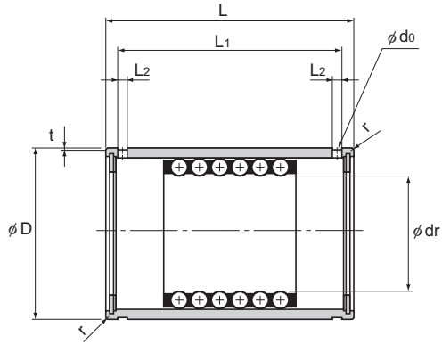
ST-B형 (중하중용)
