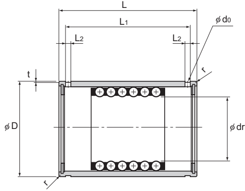
ST-B형 (中하중용)
