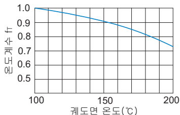
그림2 온도계수 ( f_r )
